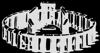
Древняя астрономическая обсерватория (Стоунхендж, Англия, II тыс. до н. э.).
