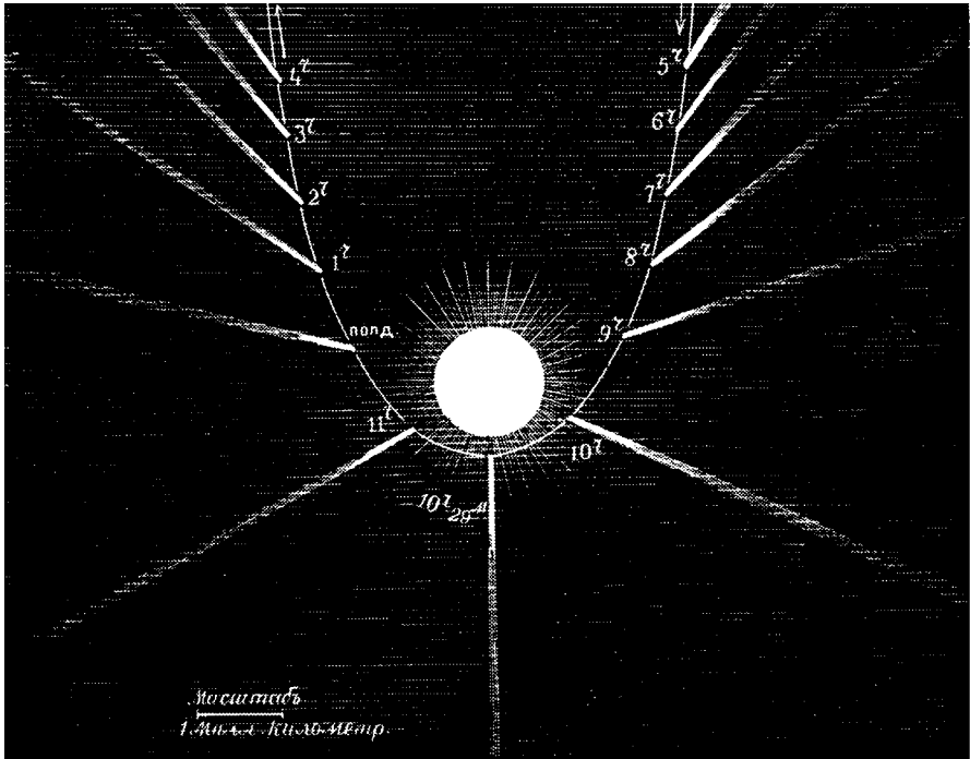
К задаче 5.97. Прохождение кометы 1843 г. вблизи Солнца 27 февраля. Вдоль траектории указано среднее парижское время.
