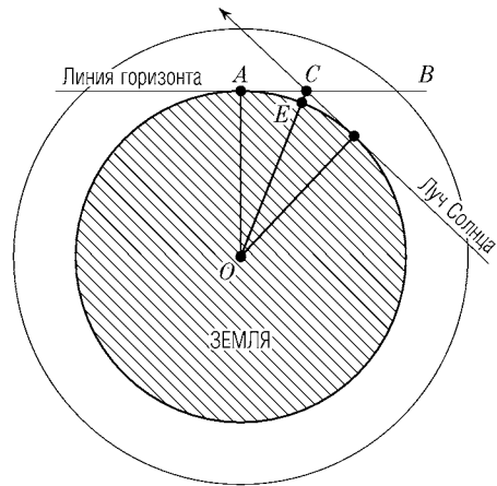
К решению задачи 5.60. Метод определения высоты атмосферы по высоте сумеречного сегмента.
