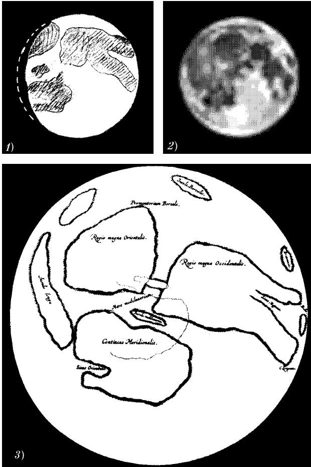
К решению задачи 4.68.
