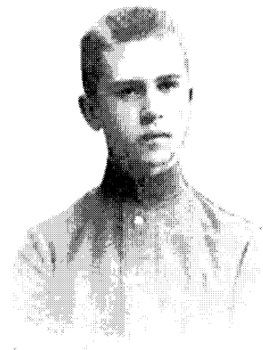
А. Борисяк, открывший Новую Персея 1901 г.
