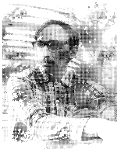
Студент МГУ Сергей Шугаров, открывший Новую Лебедя 1975 г., на фоне башии 2,6-метрового рефлектора им. Г. А. Шайна Крымской астрофизической обсерватории.
