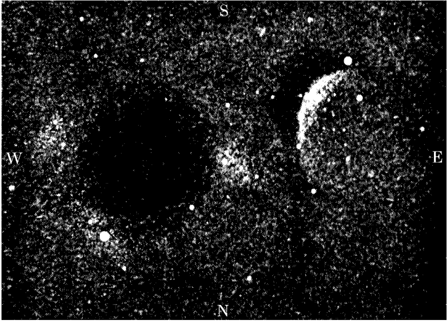
К задаче 5.12. Чёрное место в созвездии Стрельца (иллюстрация из книги Г. Клейна, 1897, с. 299).
