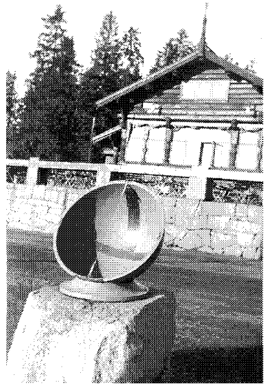
К задаче 2.4. Солнечные часы в г. Осло (фото П. Г. Куликовского, 1953 г.).
